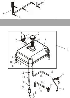
IMG. 7 SYSTÈME DE COMBUSTIBLE
