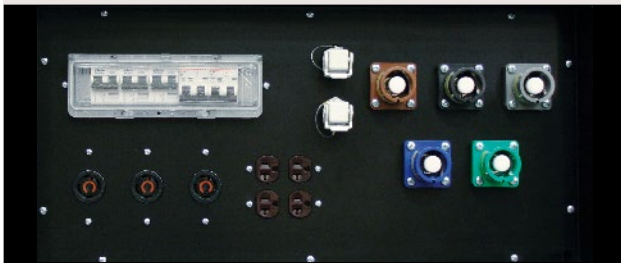
QUADRI DI DISTRIBUZIONE CON CONNETTORI 250/400/650A DISTRIBUTION PANEL WITH 250/400/650A CONNECTORS
