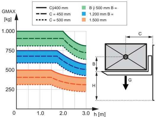
belastningskurve:
